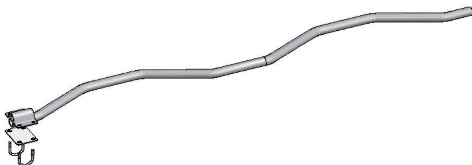
1½" zig-zag nakkerør, 2 båse 690494 c/c 109 - 111 cm 690493 c/c 114 - 116 cm 690492 c/c 119 - 121 cm 690490 c/c 124 - 126 cm 690491 c/c 129 - 131 cm inkl. bolteplade, ekskl. rørbøjler og samlerør
