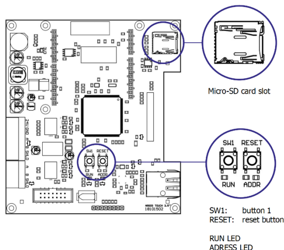
Figur 4: Frontkort layout
