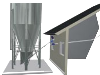
Skruvlösning B 2 Säker lösning med rörskruv till Maflexskruv. Skonsam mot fodret tack vare reglerad matning och mycket flexibelt då man har behov av foder på flera ställen i stallet. Klarar långa transportbehov.
