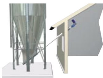
Skruvlösning B 1 En enkel och säker lösning med rörskruv till Maflexskruv. Tack vare en reglerad matning av 102 mm rörskruv till flexskruven är detta alternativ mycket skonsamt för palleterat foder vid långa transporter.
